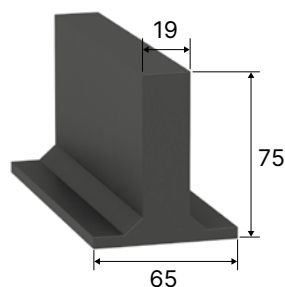
PROFILO PROFILE I
