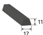
GUIDA SEZION GUIDE SECTION B
